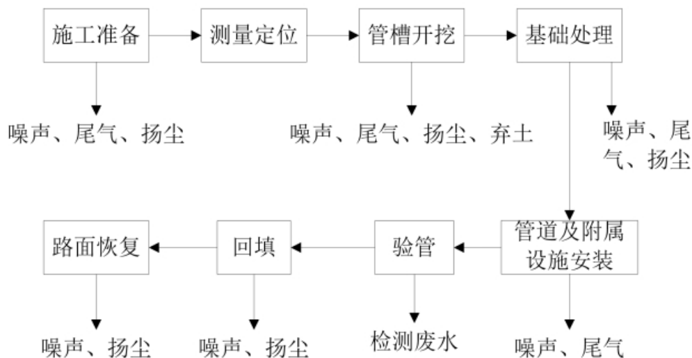
图 4-3 雨水管网施工工艺污染流程及产污环节示意图
